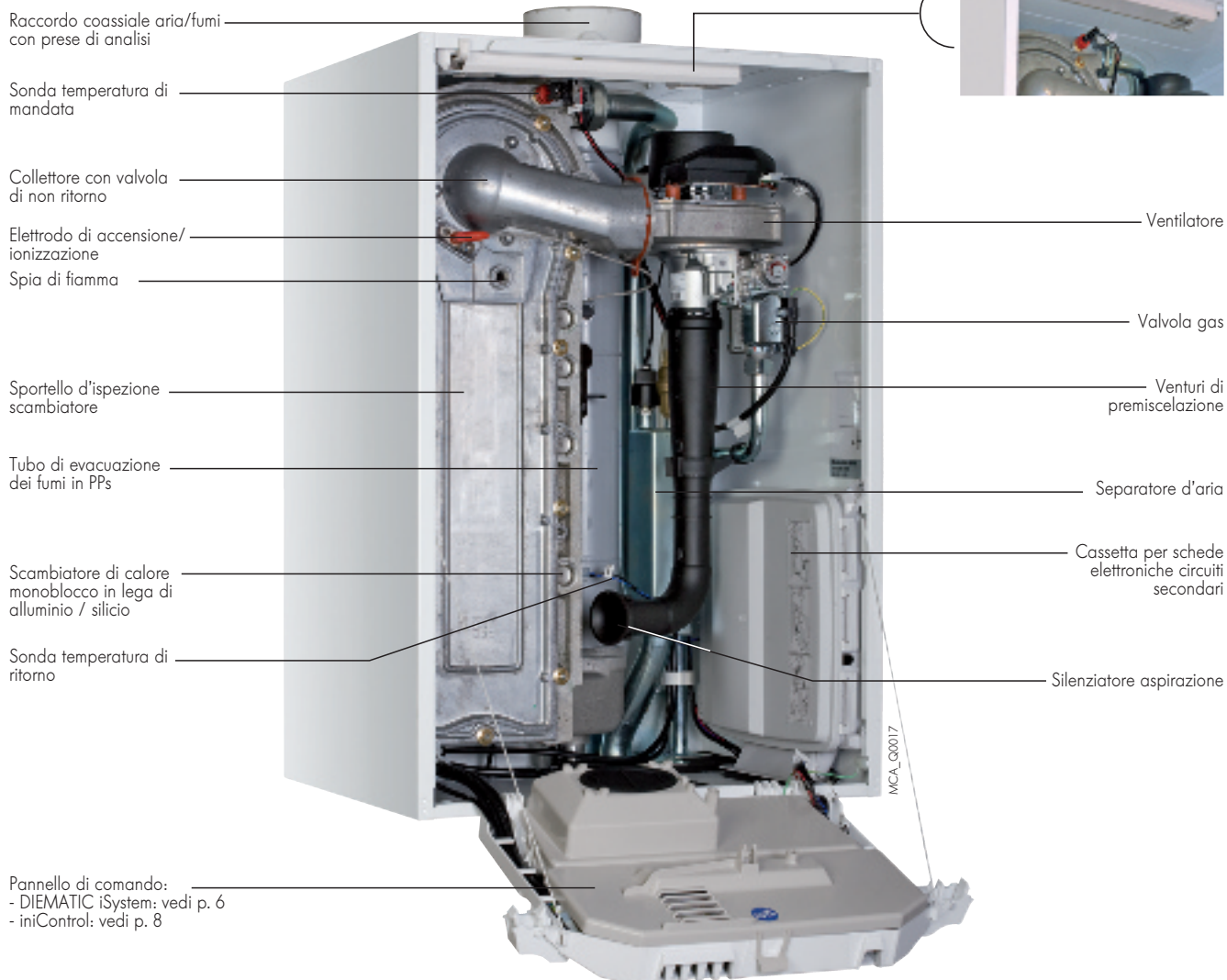
Particolari dello scambiatore di calore in lega alluminio/silicio
